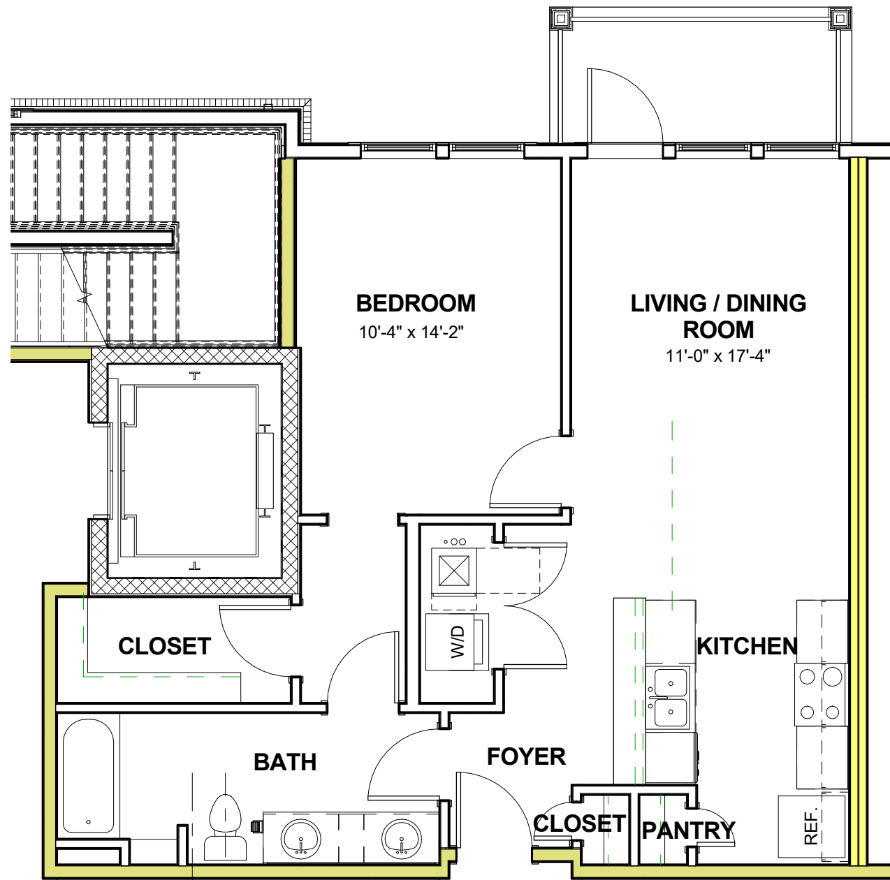
UNIT TYPE A.3 765 S.F.
